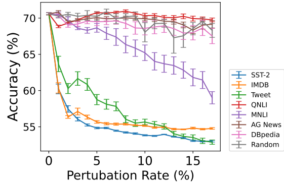
(b) On Tweet
