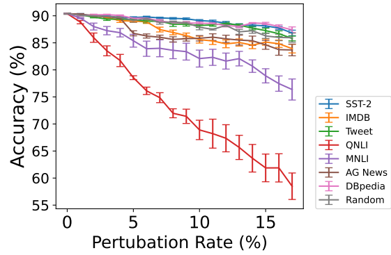
(d) On QNLI
